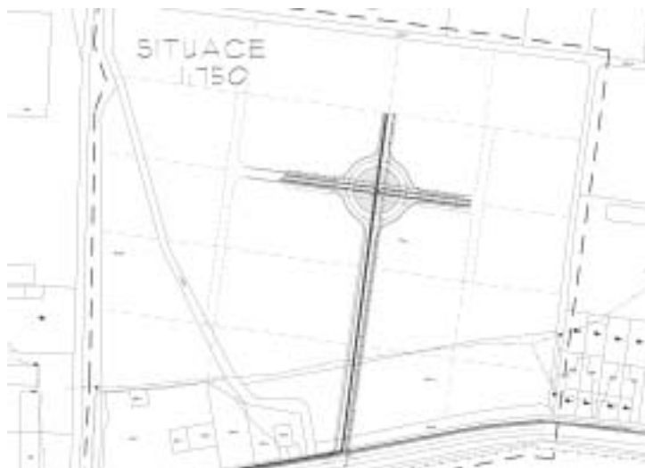
Situační plán průmyslové zóny a rozmístění inženýrských sítí.
